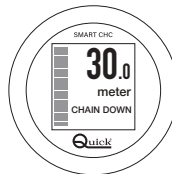
ABSSENKEN DES ANKERS (M/FT). GRÜNER BALKEN BEWEGT SICH.
